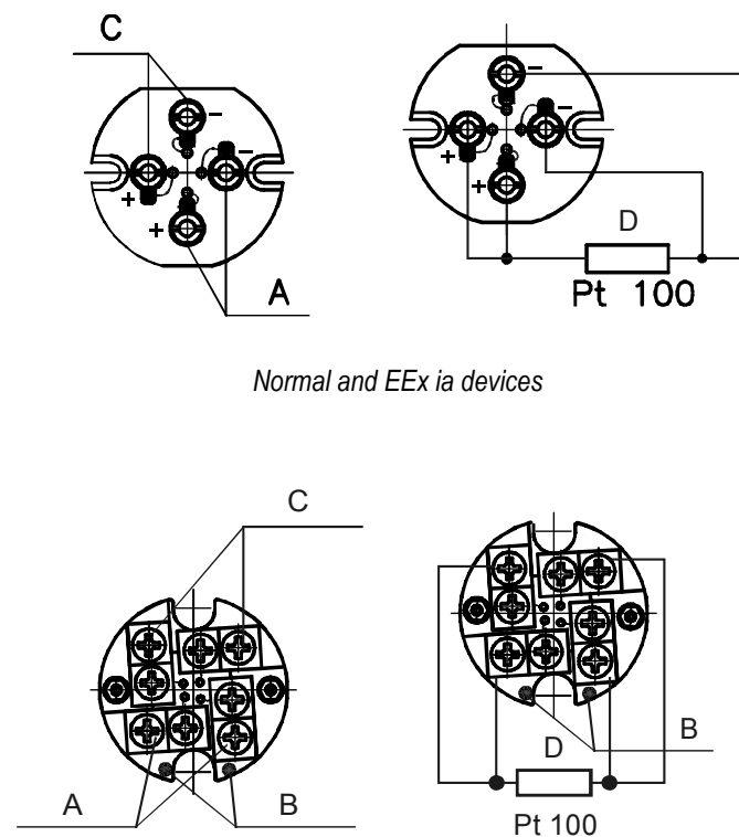
EEx d, EEx d ia devices
